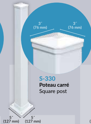
Poteaux en option pour rampes | Optional posts for railing
